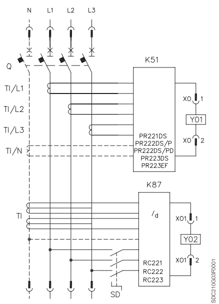
Трехполюсный или четырехполюсный автоматический выключатель с электронным распределителем защиты PR221DS, PR222DS/P или PR222DS/PD и распределителем защиты дифференциального тока RC221, RC222 или RC223 (только для четырехполюсных Т4, Т5 и Т6)
