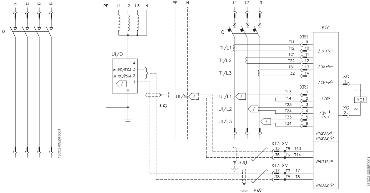
Трехполюсный или четырехполюсный выключатель-разъединитель
